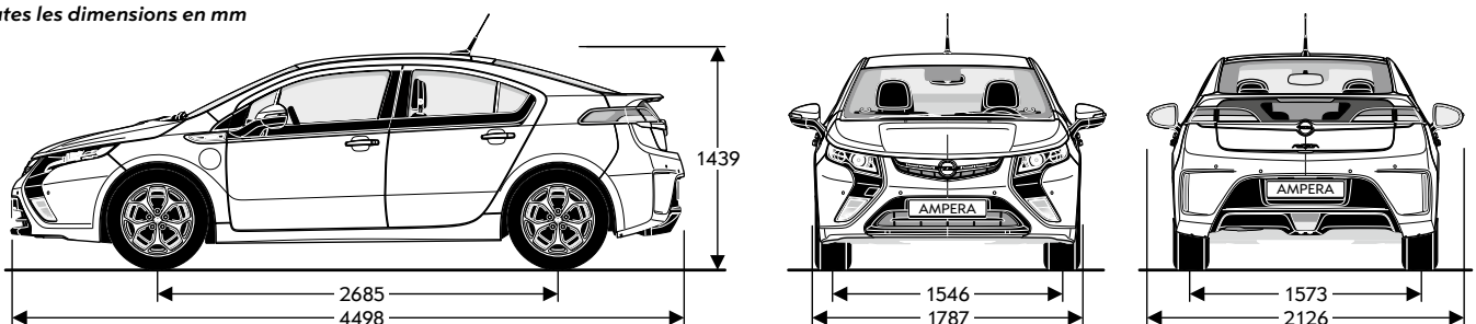
Seitenansicht 5 Türen / Côté 5 portes
